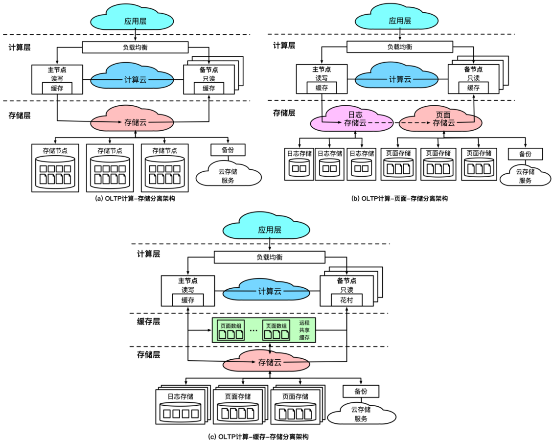
图2 云原生 OLTP 数据库三类架构设计
