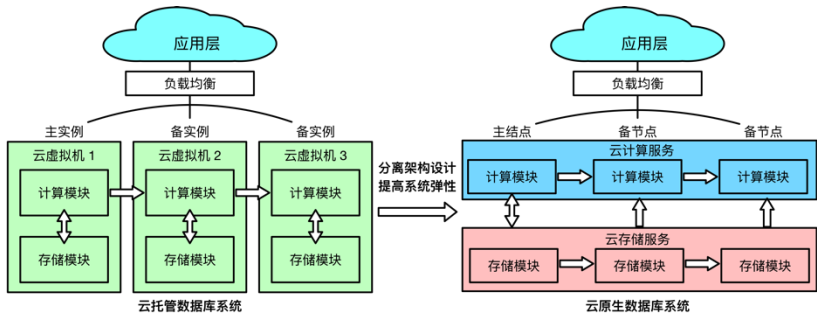
图 1 云托管与云原生数据库架构差异
