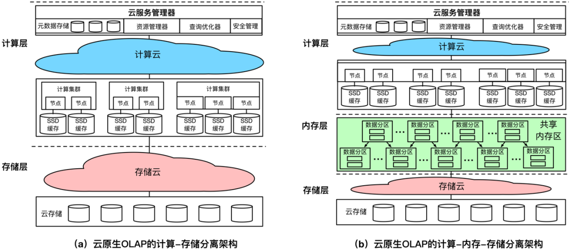
图 9 云原生 OLAP 数据库架构
