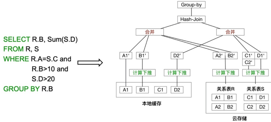
图 15 结合数据缓存与计算下推的查询处理 [44]
