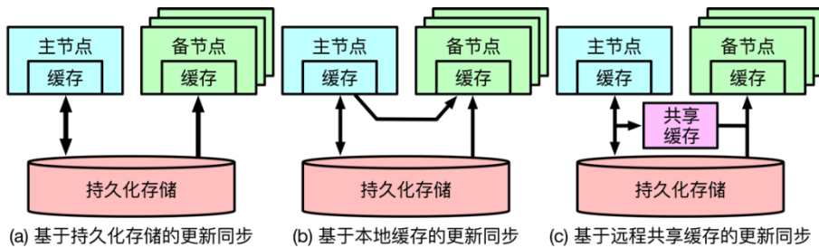
图 6 主备节点更新同步的三种方式
