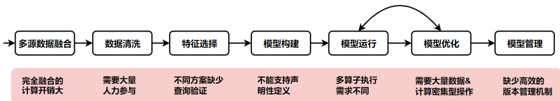
图 1 机器学习生命周期及存在的问题
